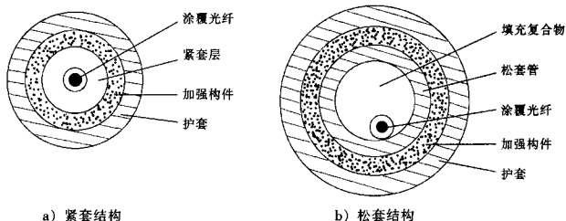
图 1 光缆结构示意图
